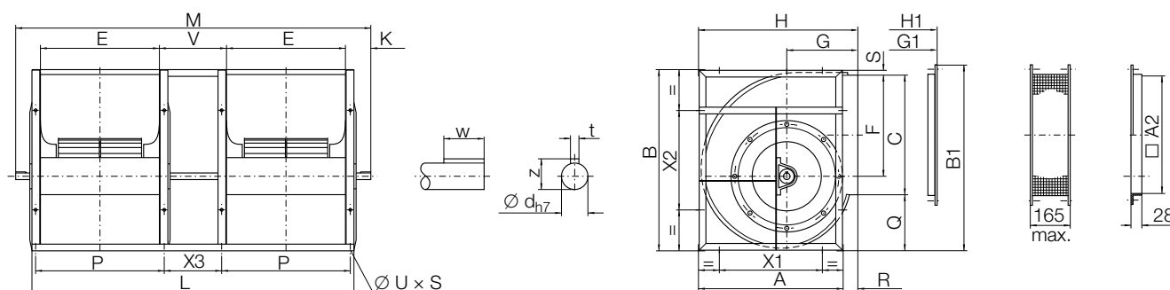
ADH G2E4-0250/-0355
